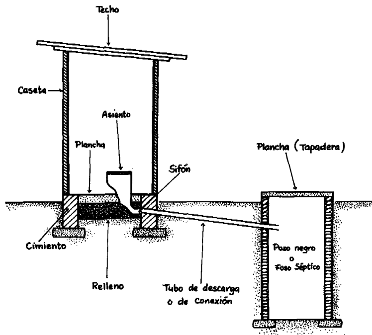
Letrina de Sello Hidráulico con descarga manual reducida
