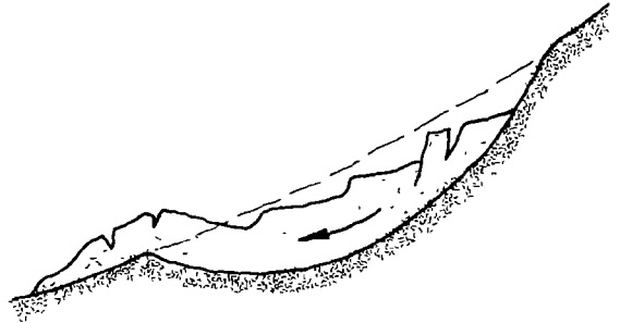
Fig. 19. A landslide
