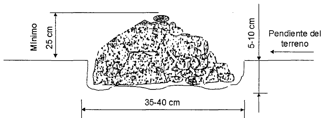
Figura 31. Bordos de piedra al contorno: Dimensiones.
