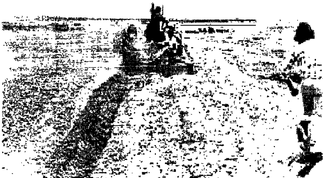
Figura 6. Arado "Xolox" para la construcción de surcos modificados (microcaptaciones), también puede ser usado con tracción animal.
