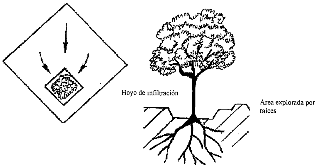
Figura 12. Sistema de microcaptación negarim para árboles.
