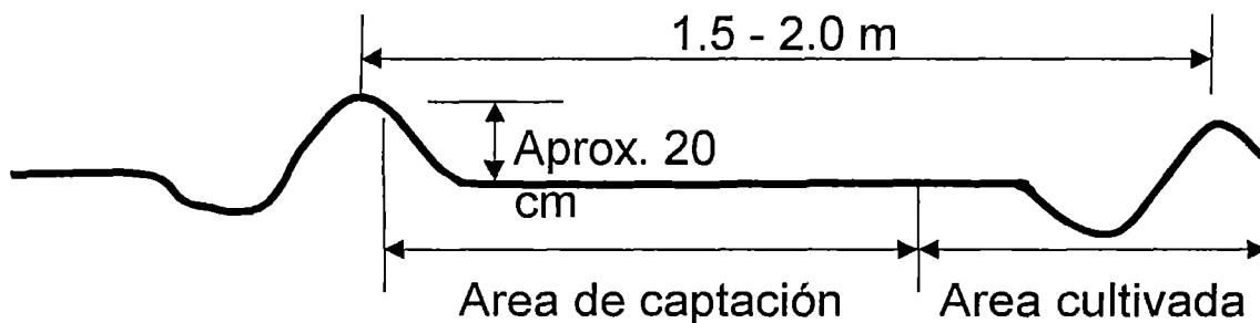
Figura 15. Dimensiones de camellones y surcos en contorno.
