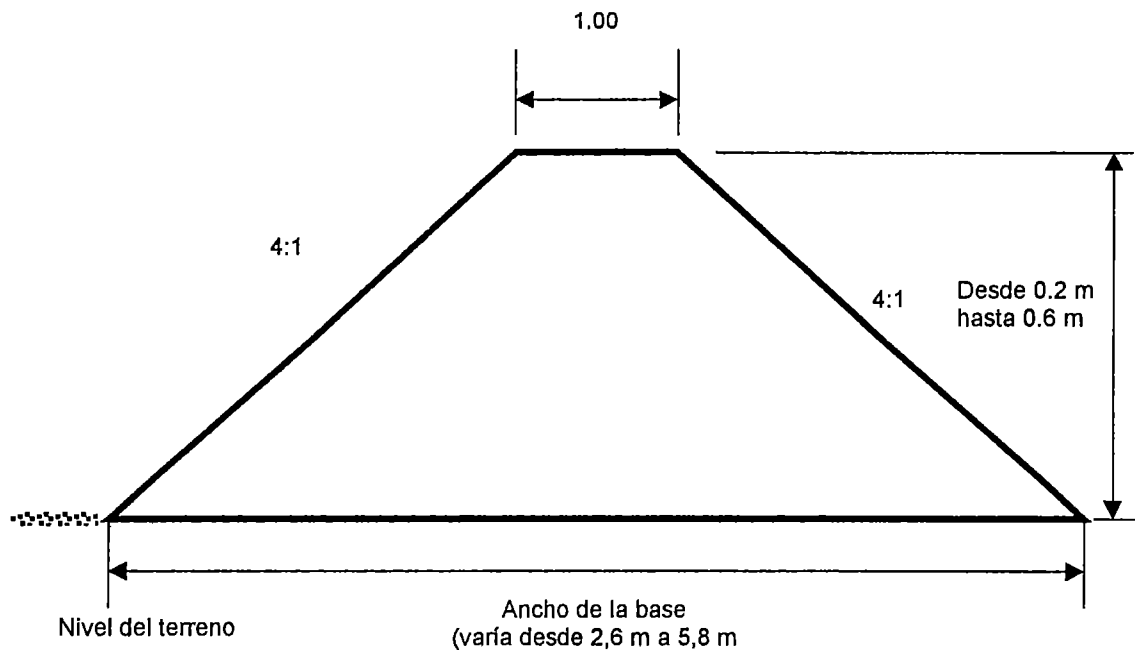
Figura 22 . Bordos Trapezoidales: Sección transversal.
