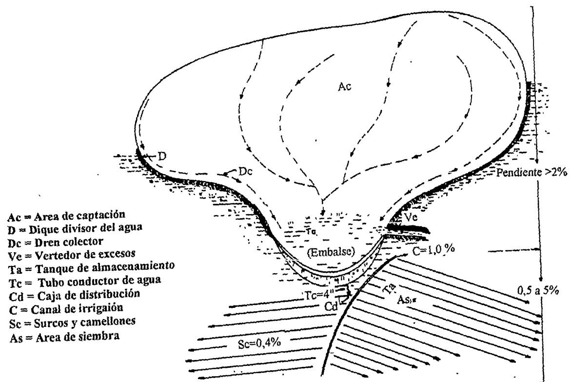
Figura 42. Modelo esquemático del sistema de aprovechamiento de escorrentía superficial en embalses.
