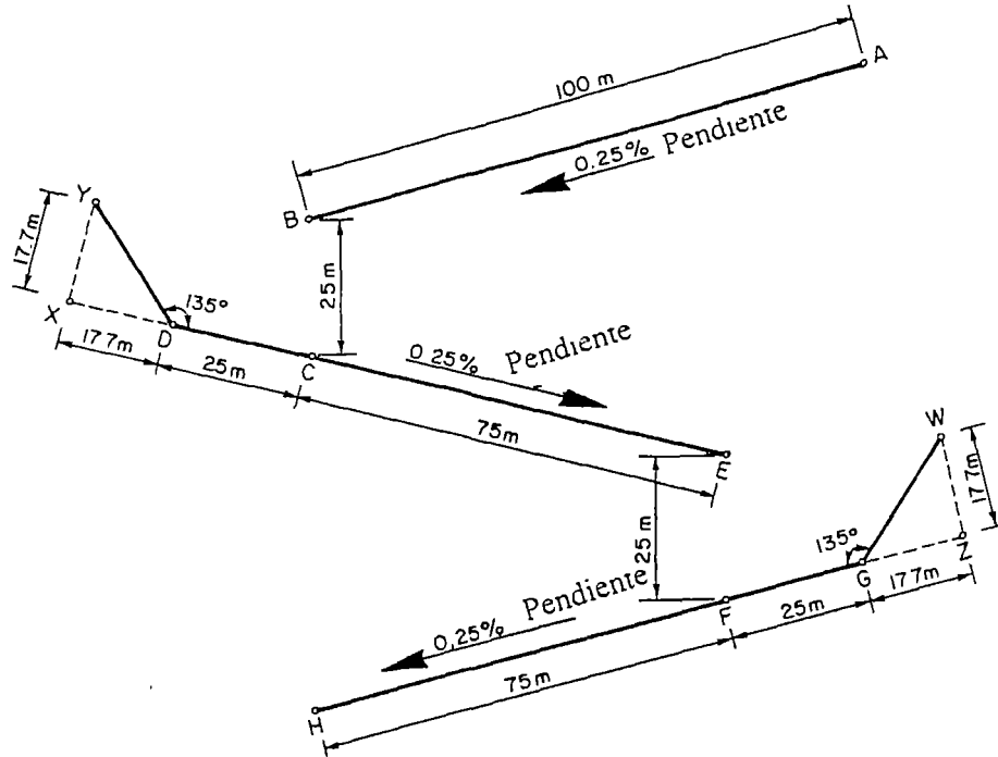
Figura 40. Establecimiento del bordo escalonado: para pendientes > 0.5\% .
