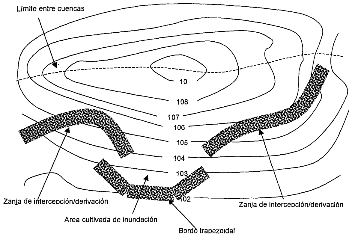
Figura 28. Zanjas de intercepción.
