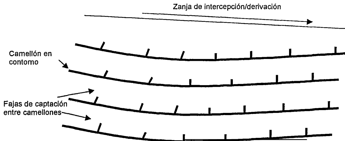
Figura 14. Camellones y surcos en contorno: esquema de campo.
