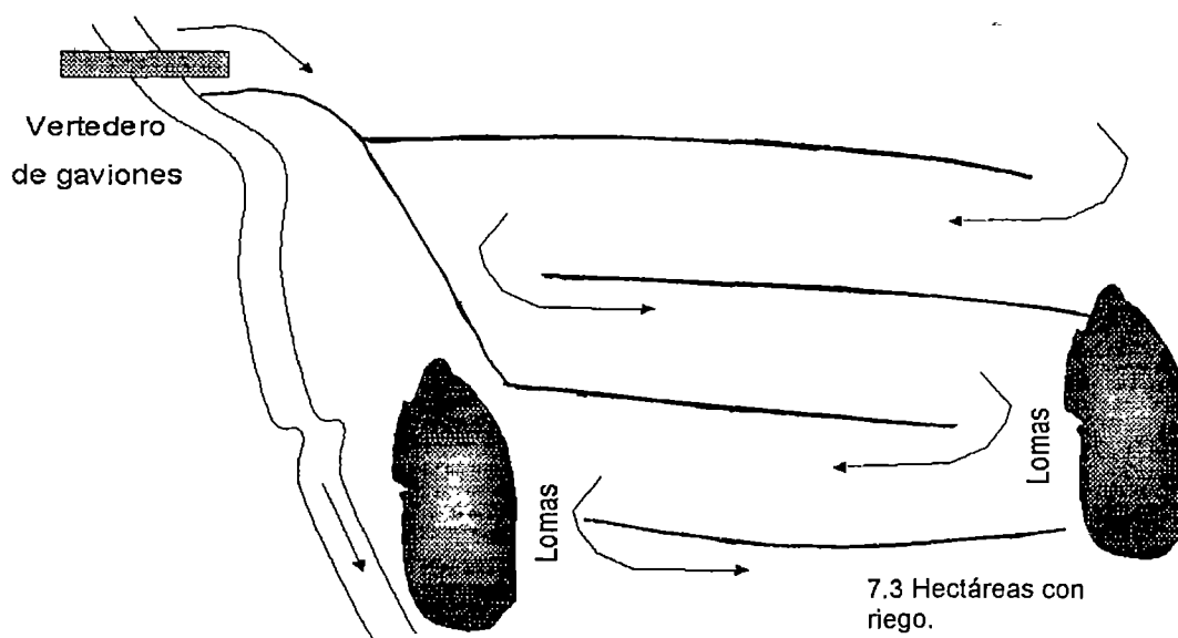
Figura 38. Esquema piloto IMPALA sobre dispersores de agua en Turkana, Kenya.
