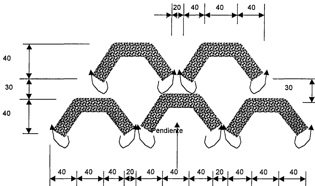
Figura 20. Bordos trapezoidales: trazo de campo para pendientes del terreno de 1%.
