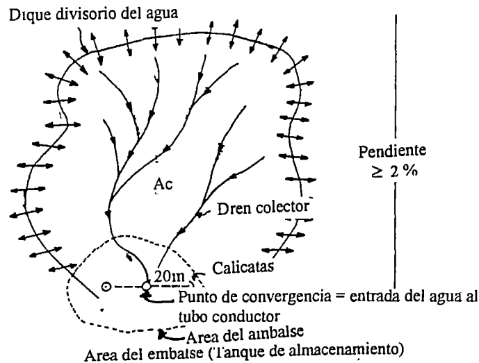
Figura 43. Localización del Área de Captación (Ac) y del Tanque de Almacenamiento (Ta) con relación al punto de convergencia natural de las aguas de escorrentía.
