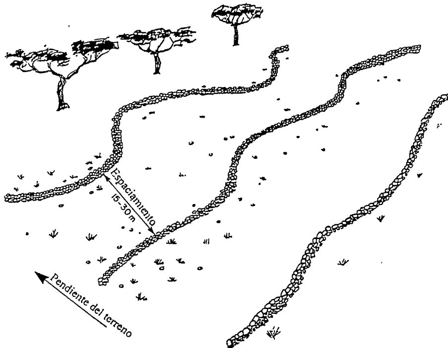
Figura 30. Bordos de piedra el contorno: Trazo en campo. (Fuente: Critchley y Reij, 1989).
