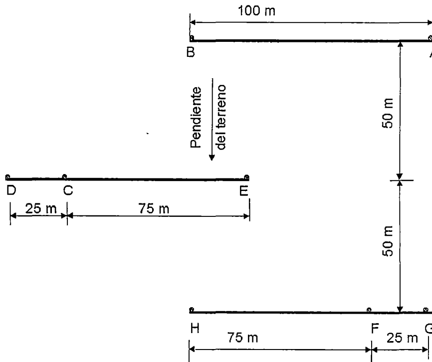
Figura 39. Trazo de bordos a nivel: pendiente < 0,5%.
