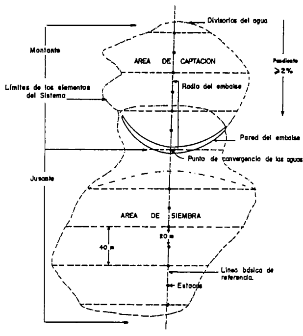
Figura 46. Modelo esquemático de la localización de los elementos básicos del SAES-ES, en campo.
