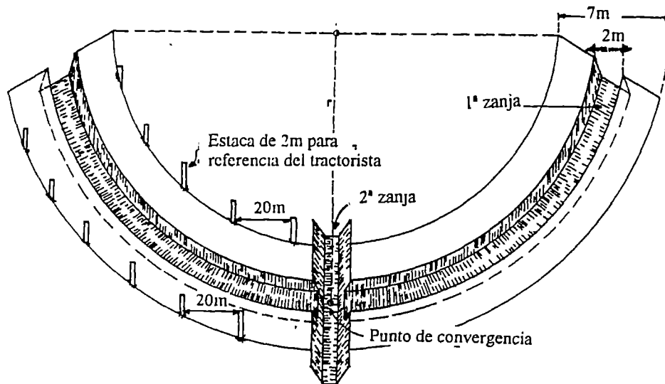
Figura 47. Modelo esquemático de las zanjas que servirán de fundación para la pared del embalse y para la instalación del tubo conductor del agua.
