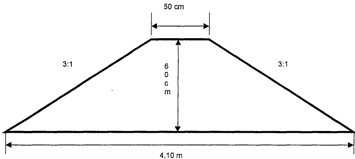
Figura 36. Dimensión de bordos.
