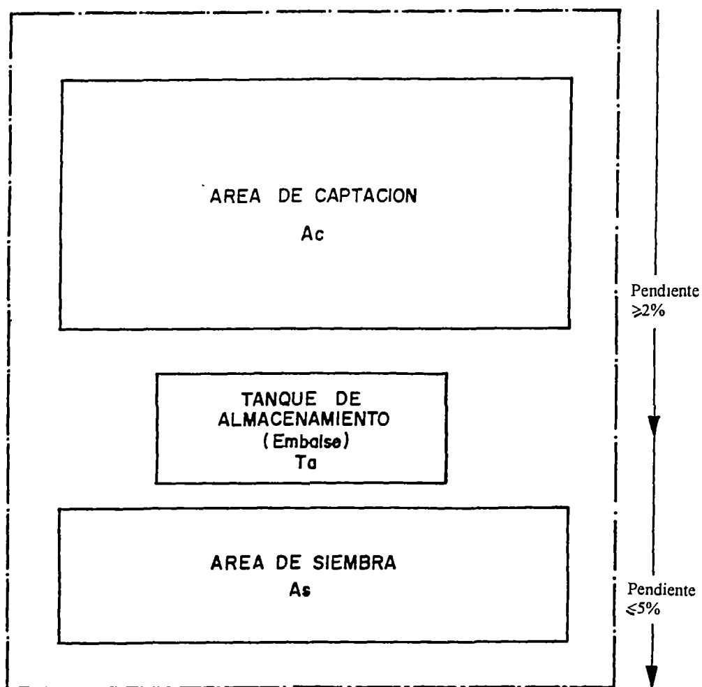
Figura 44. Disposición espacial de los elementos básicos del SAES-UA.
