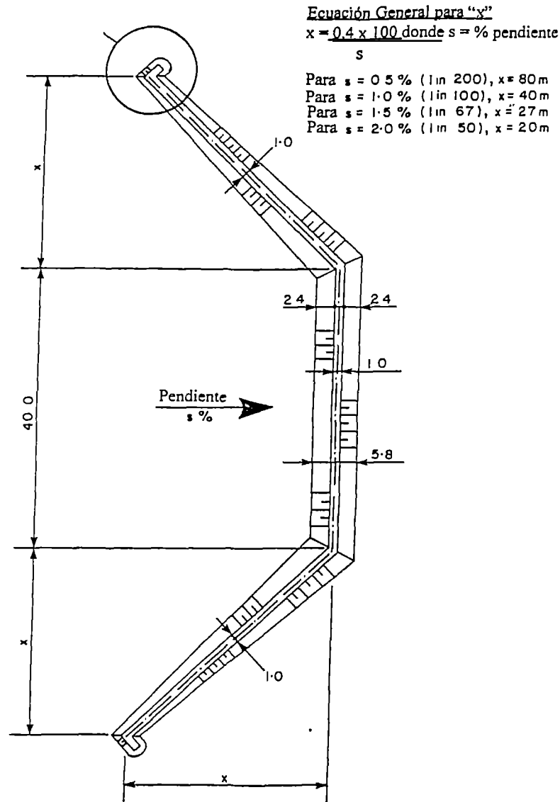
Figura 21. Dimensiones de bordos trapezoidales.
